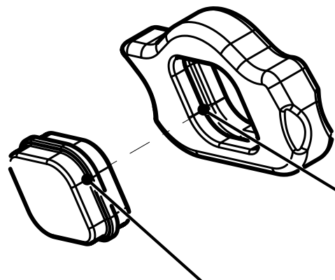
Inneres Elastomer - Austauschbar zum Einstellen auf das Fahrergewicht
